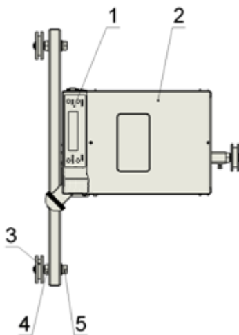
1—Панель управления; 2—Блок измерительный; 3—Колесо; 4—Ось-эксцентрик; 5—Болт
